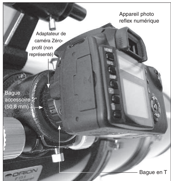
Figure 6. La fixation d'un appareil photo reflex numérique nécessite une bague en T compatible avec le modèle particulier d'appareil photo et d'un adaptateur en T, comme l'Orion Zero-Profile Prime Camera Adapter Focus, qui s'insère dans le collier de 2" (50,8 mm).
