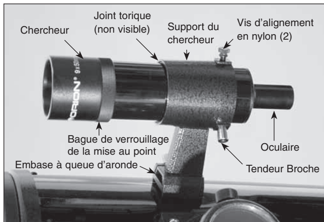
Figure 3a. Le chercheur 9x50 et son support
